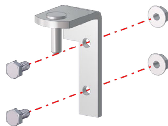
Fig. 60: Remove Bottom Hinge
